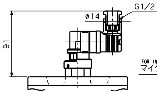
VARIOUS PARTS DIMENSION & STANDARD FLOW RATE 各部寸法並びに標準流量表
